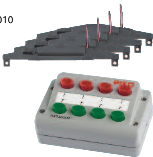
55392 Weichenantrieb-Set Set aus Stellpult 55262 zum Schalten von Weichen oder Signalen und 4 elektrischen Weichenantrieben 55271
