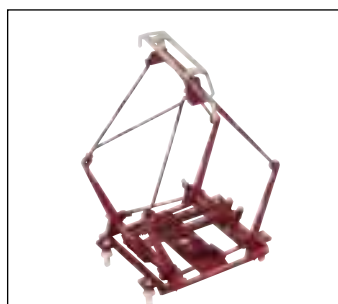
6074 Confezione 2 pantografi FS 52/92 con strisciante piano. Box of 2 FS 52/92 pantographs.
