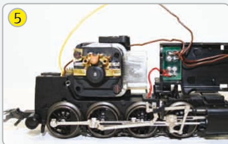
5 Montieren Sie das Motorschild wieder vorsichtig: Die Kohlebürsten dabei leicht anheben bzw. auseinanderziehen, damit sich das Motorschild über dem Kommutator montieren lässt.
