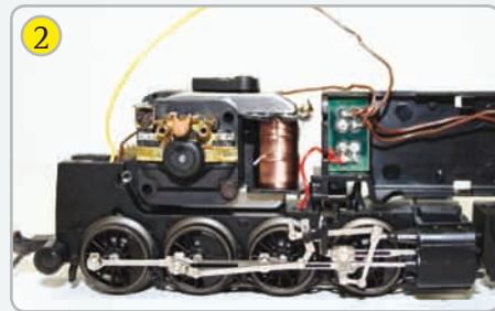
2 Allstrommotor mit angeschl. Delta-Decoder. Entfernen Sie alle Drähte zwischen Motor und Decoder und alle Entstörkondensatoren außer dem zwischen den Motoranschlüssen.
