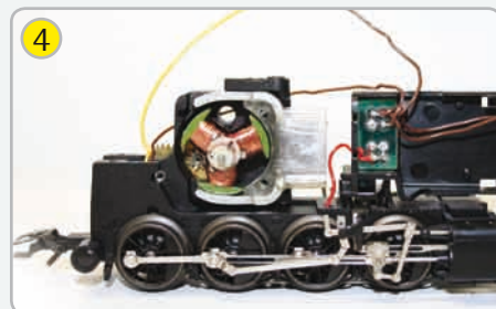
4 Ziehen Sie die alte Feldspule ab und ersetzen Sie sie durch den passenden Permanentmagneten.
