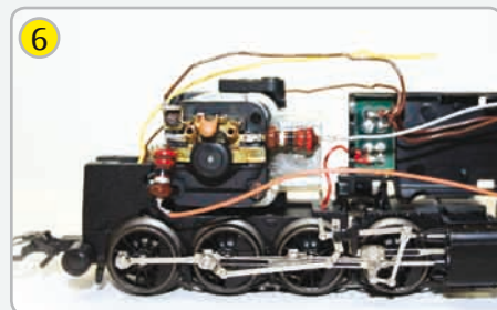
6 Löten Sie an jeden Motoranschluss eine Entstördrossel und verbinden Sie das andere Ende mit dem grauen bzw. orangenen Kabel des LokPilot bzw. LokSound Decoders. Fertig ist Ihr Motorumbau!
