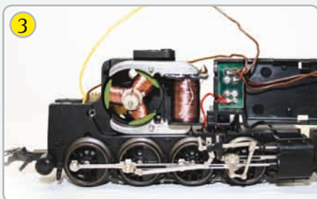
3 Entfernen Sie die beiden Schrauben am Motorschild und heben Sie das Motorschild vorsichtig ab. Achten Sie darauf, dass die Kohlebürsten nicht verloren gehen!
