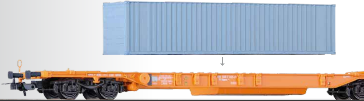
Doppeltragwagen Sdggmrs 744 „Kombiwaggon“ der DB AG, beladen mit zwei 20" Container „Hapag Lloyd“ und einem 40" Container „China Shipping“ / Container car Sdggmrs 744 of the DB AG with two 20" containers „Hapag Lloyd“ and one 40" container „China Shipping“
