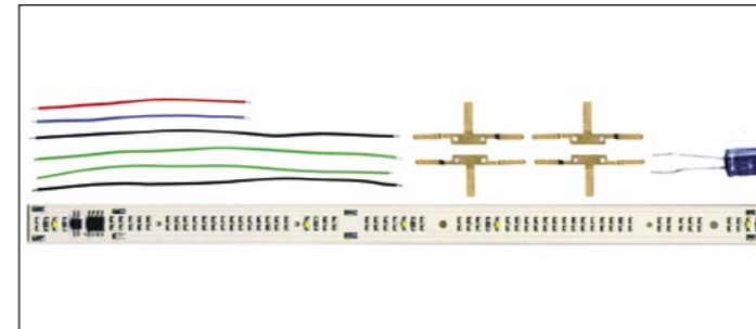
6075 Confezione contenente kit di illuminazione per la carrozza delle FS. Lighting kit for passenger coach of the FS.
