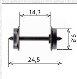
6049 Set 4 assali Ø 9,8 mm. Set 4 axles Ø 9,8 mm.
